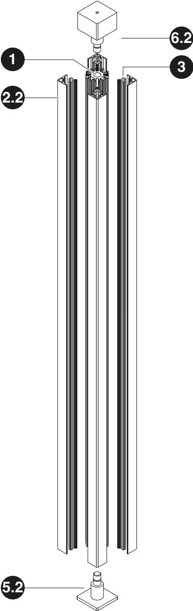
Applicazione a soffitto / Ceiling application
