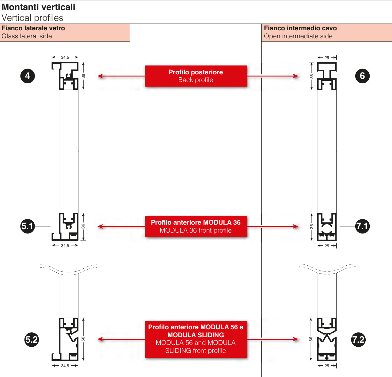
Composizione dei fianchi - vista dall'alto Sides composition - top view
