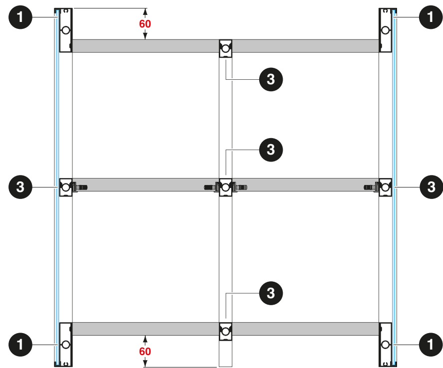
Composizione del mobile - vista frontale Cabinet composition - front view
