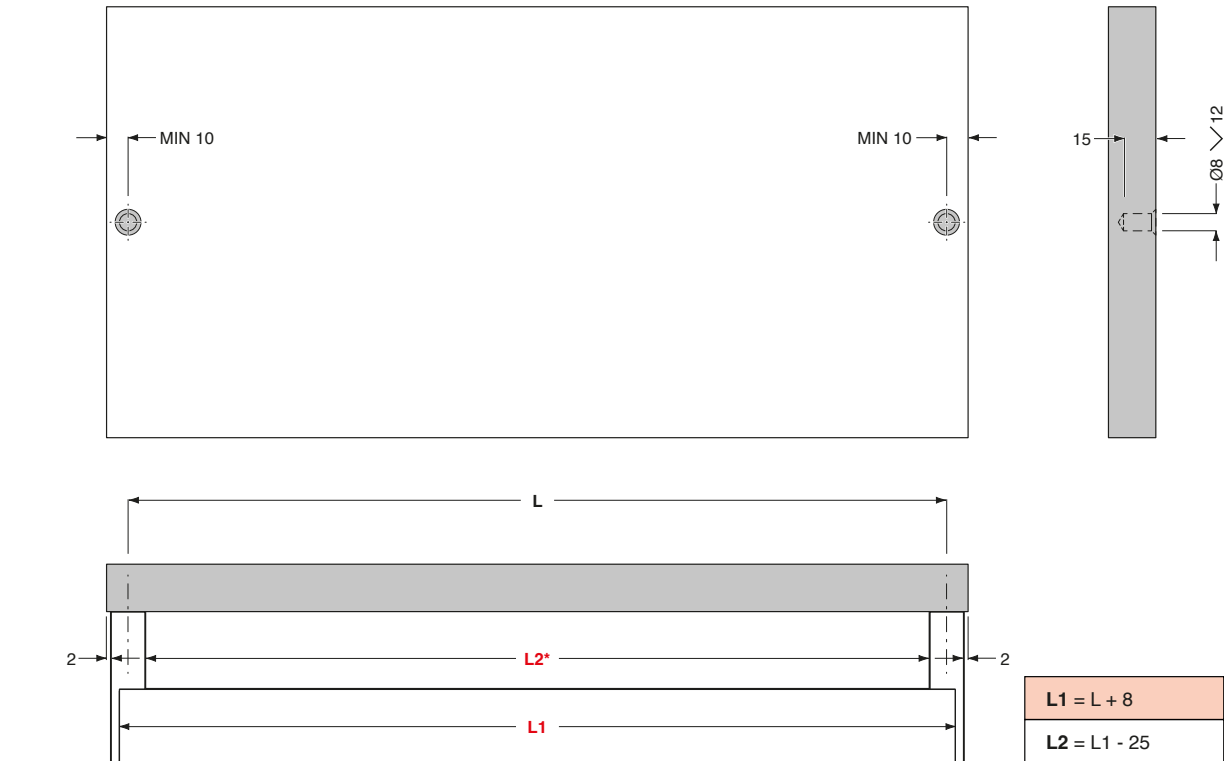
*Lunghezza guarnizione per tubo appendiabiti - Gasket for aluminium rod for clothes hanger
